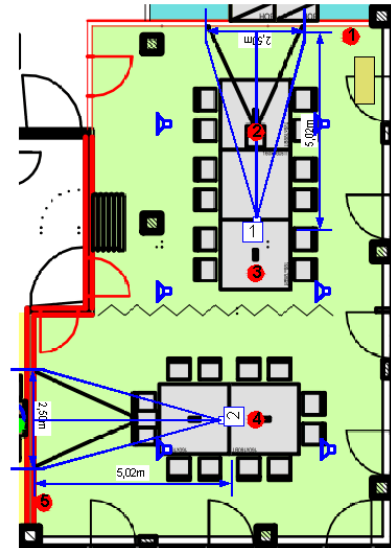
Planungsskizze für Audio-Video-Technik im Konferenzraum
